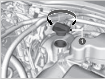
1 Oliepåfyldningsdæksel
