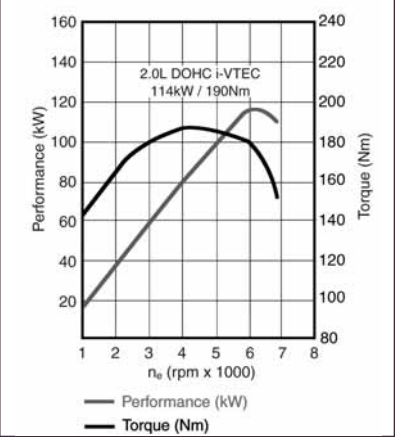
Effekt- og drejningsmomentdiagram for 2,0-liters motoren.
