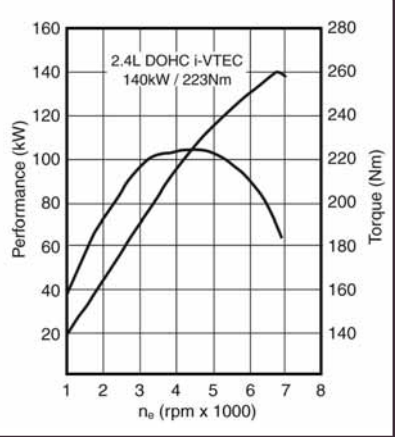
Effekt- og drejningsmomentdiagram for 2,4-liters motoren.
