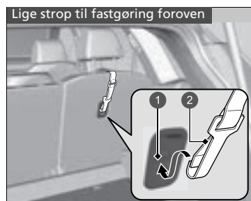
1 Befæstningspunkt
