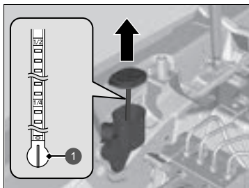
1 Væskemåler
