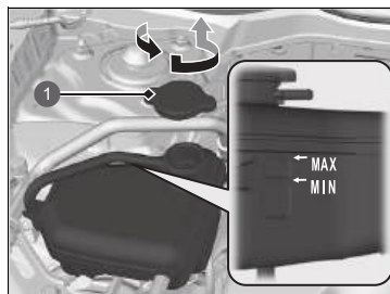
① Dæksel til reservetank
