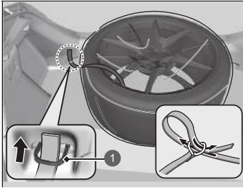
1 Bageste befæstningspunkt
