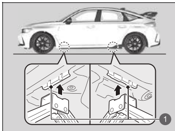
1 Løftepunkter
