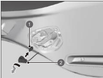
1 Pære
